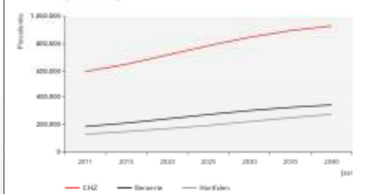
Figuur 3.1 Toename in aantal patiënten met chronische hartziekten (CHZ) met behuure en leeftijd in de periode 2011-2040: degressie en verspreiding voor de Nederlandse bevolking (basisgegevens)
